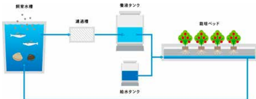
「アクアポニクス」の仕組み
